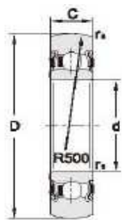
LR6...NPPU
